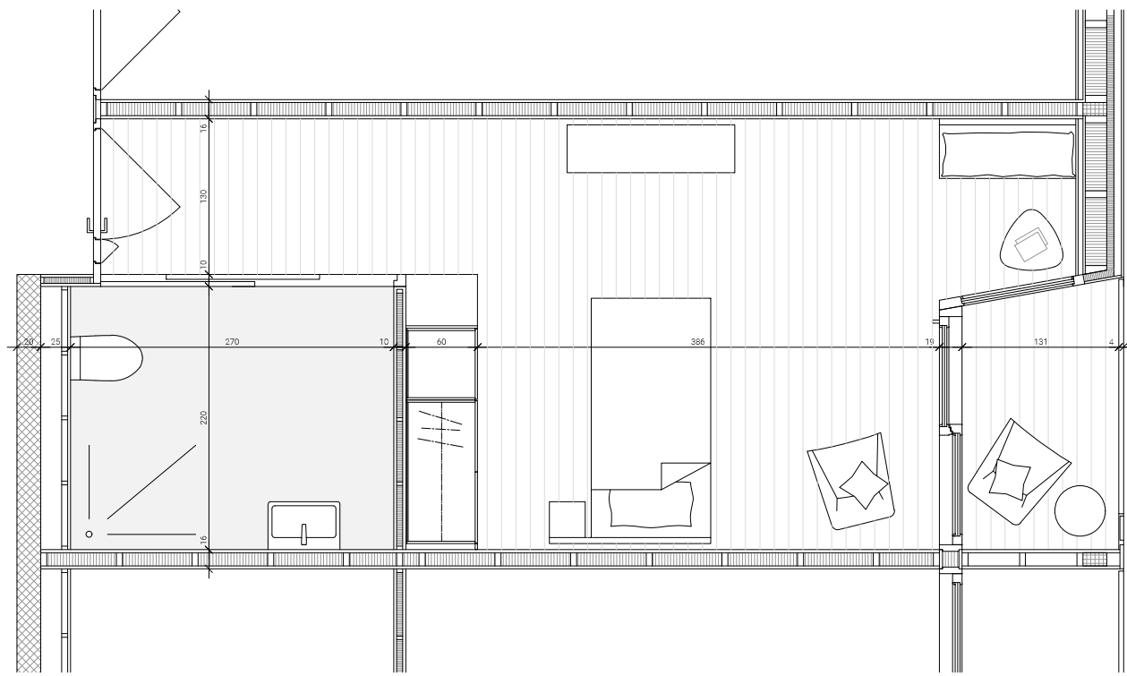
CHAMBRE TYPE 1:20
